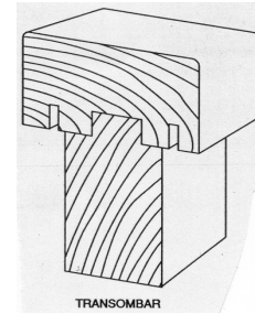
TRANSOMBAR
